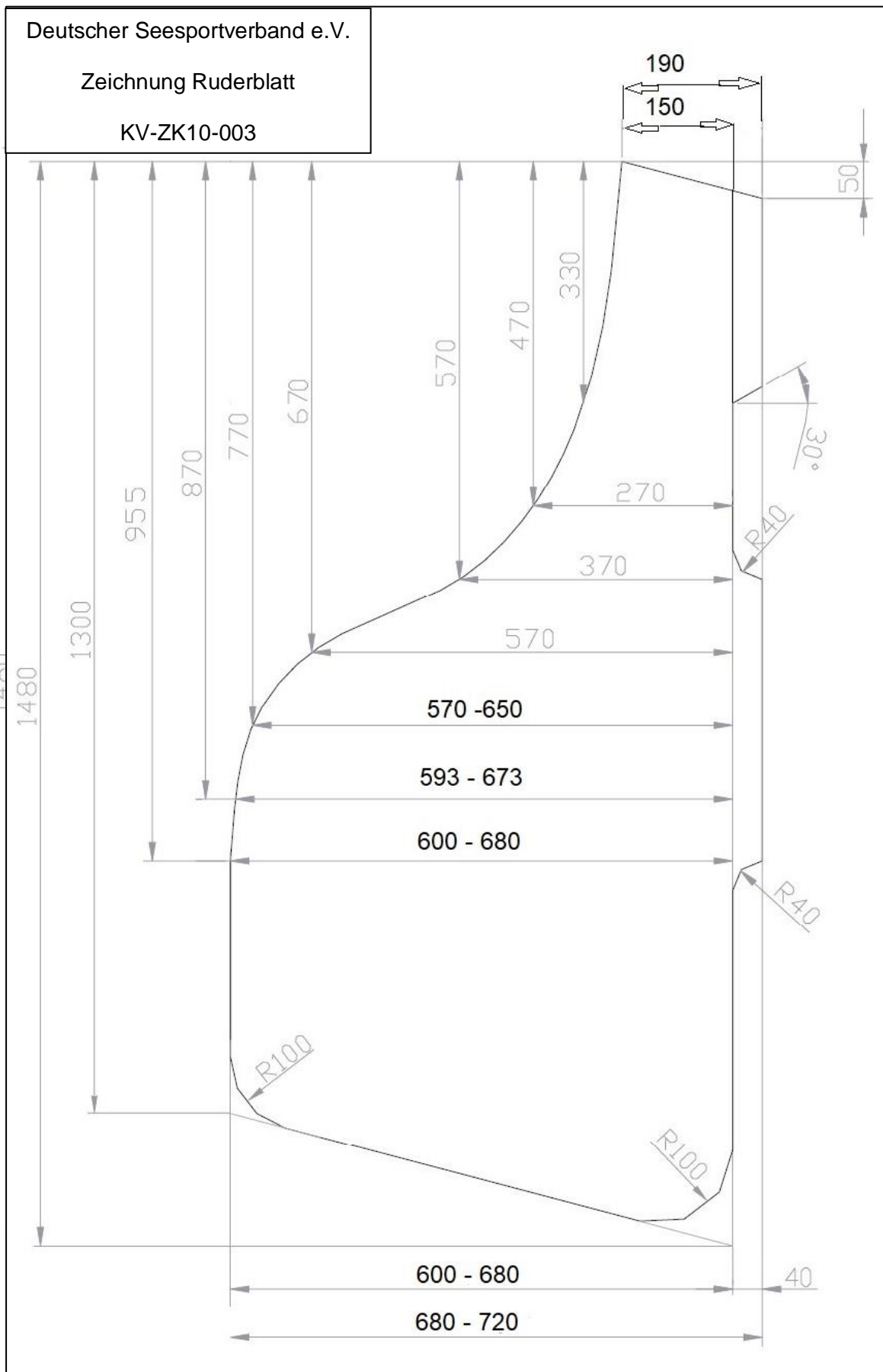
Abbildung 12 - Zeichnung Ruderblatt KV-ZK10-003
