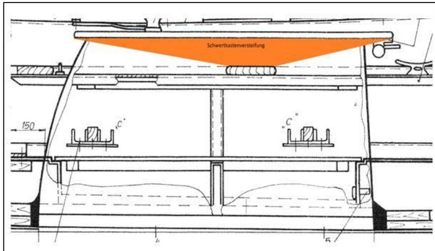
Abbildung 5 - Versteifung von der 1. Arbeitsducht aus, über die gesamte Länge des Schwertkastens nach Zeichnung KV-ZK10
