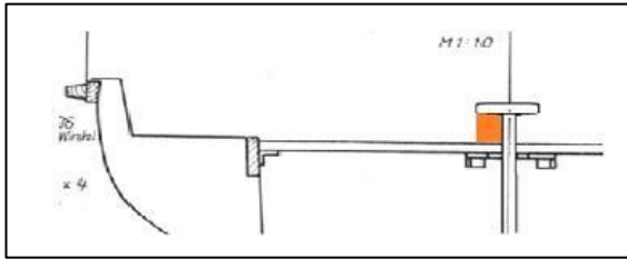
Abbildung 6 - Knie auf der 1. Arbeitsducht nach Zeichnung KV-ZK10
