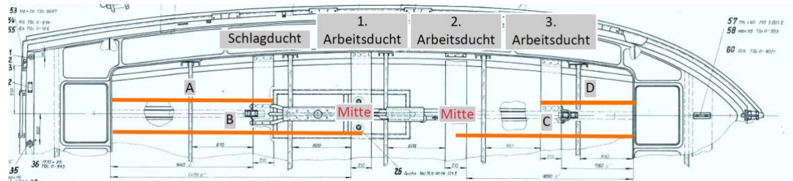
Abbildung 3 - Auszug aus Zeichnung KV-ZK10-005
