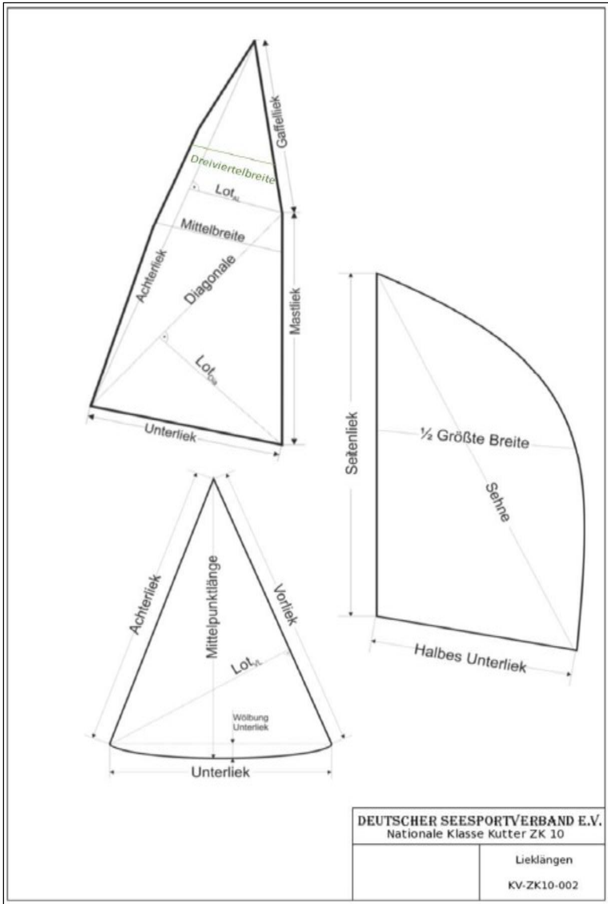
Abbildung 10 - Lieklängen Zeichnung KV-ZK10-002
