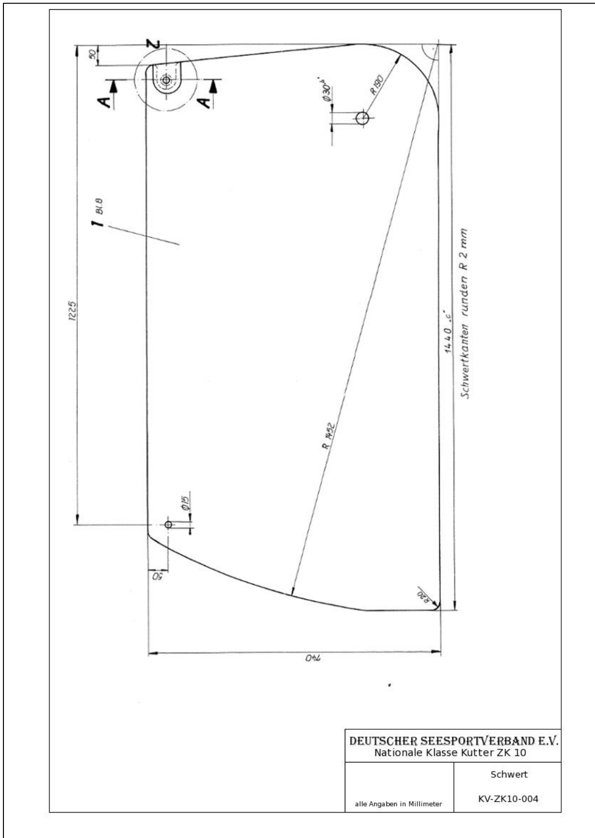
Abbildung 13 - Zeichnung Schwert KV-ZK10-004
