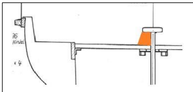
Abbildung 4 - Kantholz auf der 1. Arbeitsducht nach Zeichnung KV - ZK 10
