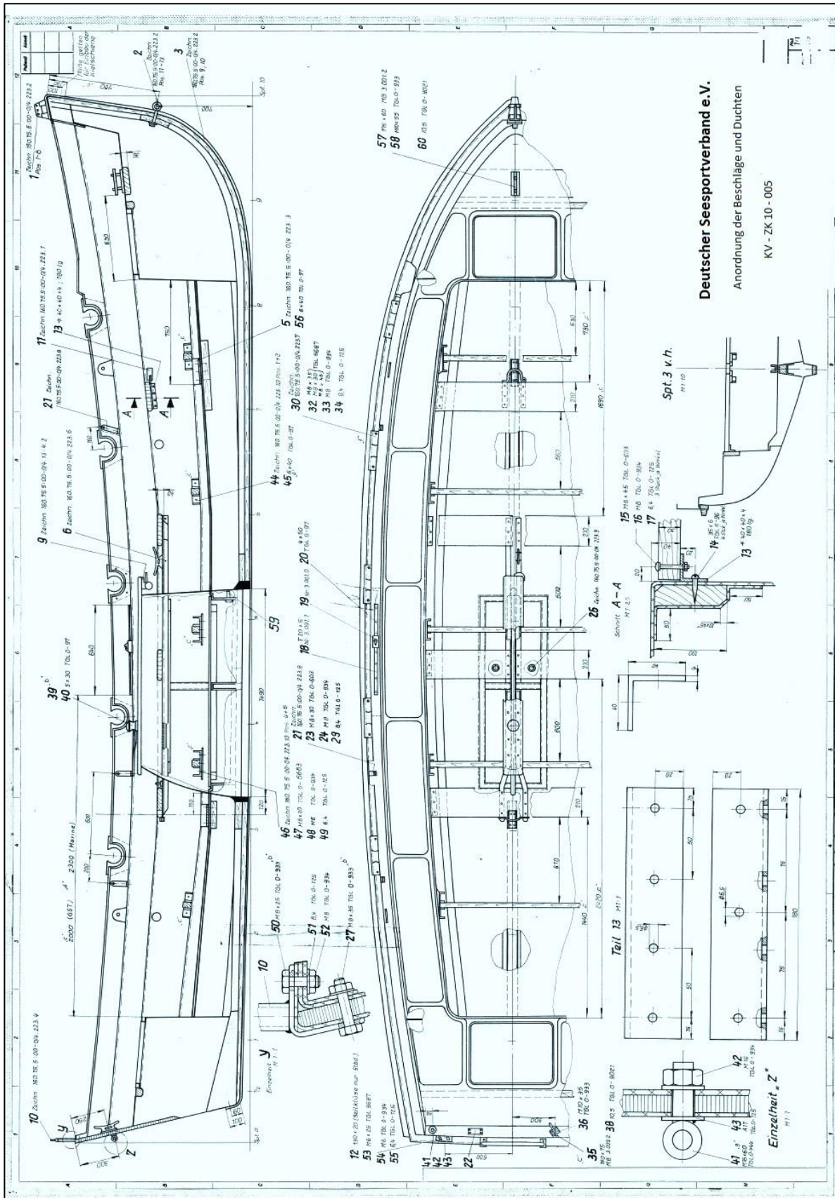
Abbildung 14 - Zeichnung Anordnung der Beschlage und Duchten KV-ZK10-005
