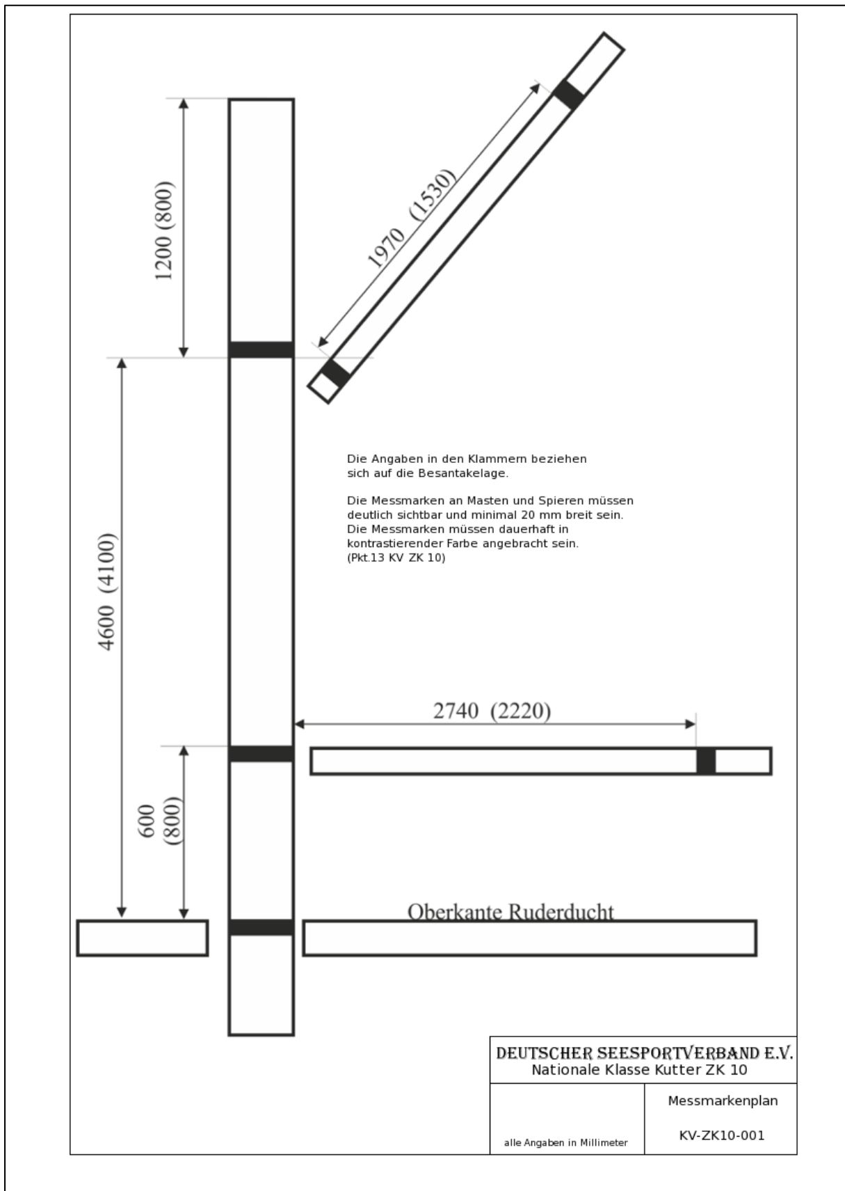
Abbildung 11 - Messmarkenplan
