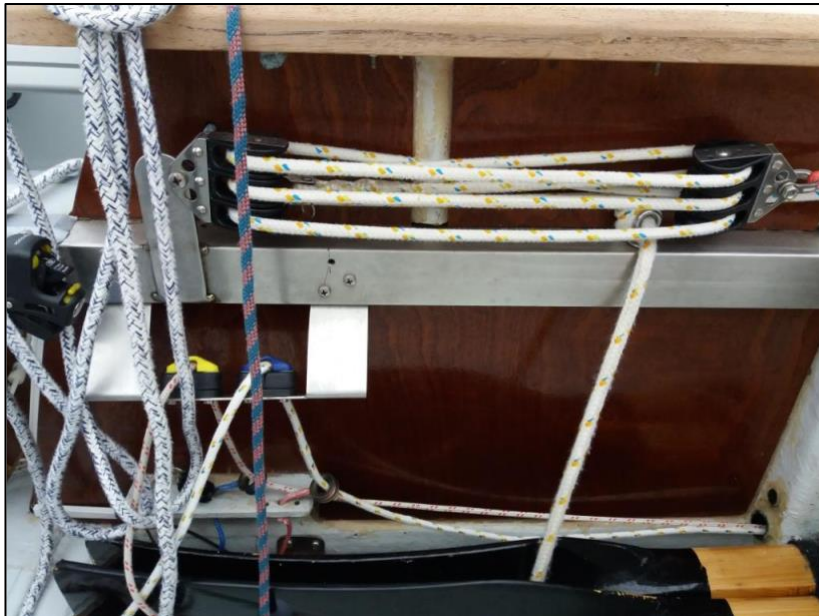
Abbildung 9 - Schwertkasten mit Sperrholz - Bild 3
